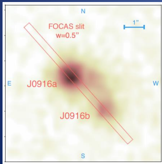
すばる望遠鏡の広視野探査で見つかった宇宙初期の活動銀河中心核の例(左 Akiyama et al. 2018) 宇宙初期の銀河分布(色マップ)と活動銀河中心核の分布(赤星印)の比較(右 He et al. 2018)
