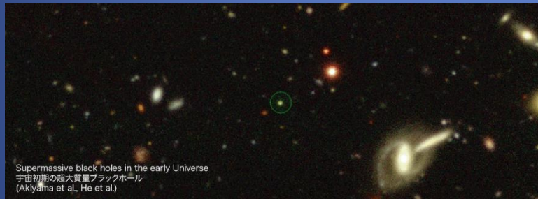
すばる望遠鏡の広視野探査で見つかった宇宙初期の活動銀河中心核の例(左 Akiyama et al. 2018) 宇宙初期の銀河分布(色マップ)と活動銀河中心核の分布(赤星印)の比較(右 He et al. 2018)
