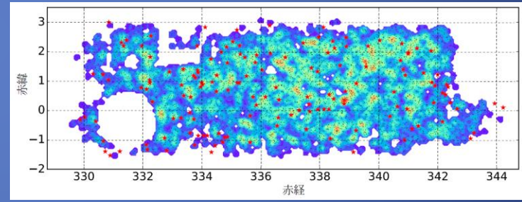
すばる望遠鏡の広視野探査で見つかった宇宙初期の活動銀河中心核の例(左 Akiyama et al. 2018) 宇宙初期の銀河分布(色マップ)と活動銀河中心核の分布(赤星印)の比較(右 He et al. 2018)
